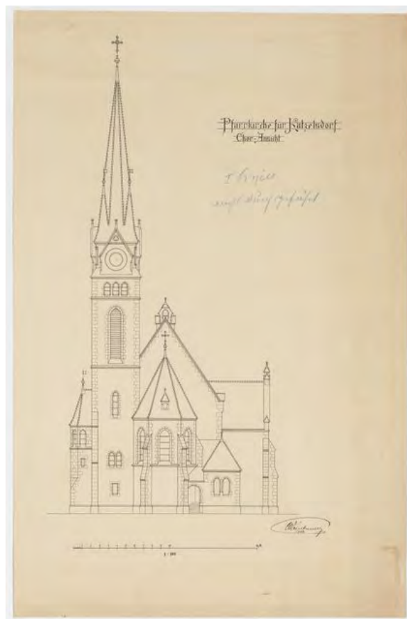
sign_6871 ... Pfarrkirche für Katzelsdorf / Chor-Ansicht / „I Projekt nicht durchgeführt“ / 1:100 / CW 1902
