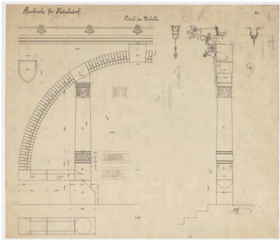
sign_6922 ... Pfarrkirche für Katzelsdorf. / 53. / Detail der Vorhalle. / 1:10 / CW 1905
