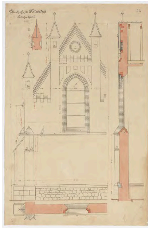
sign_6917 ... Pfarrkirche für Katzelsdorf. / 49. / Seitliche Giebel. / o. D.
