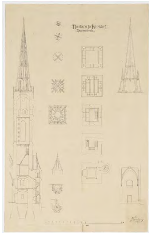
sign_6874 ... Pfarrkirche für Katzelsdorf / Thurmschnitte / 1:100 / CW fstl. Architekt 1902
