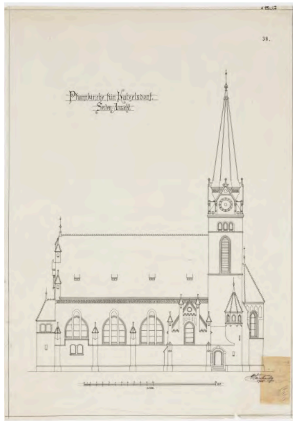
sign_6895 ... Pfarrkirche für Katzelsdorf. / 38. / Seiten-Ansicht. / 1:100 / CW 1905
