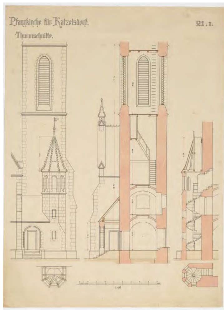
sign_6882 ... Pfarrkirche für Katzelsdorf. / 21. a. / Thurmschnitte. / 1:50 / o. D.
