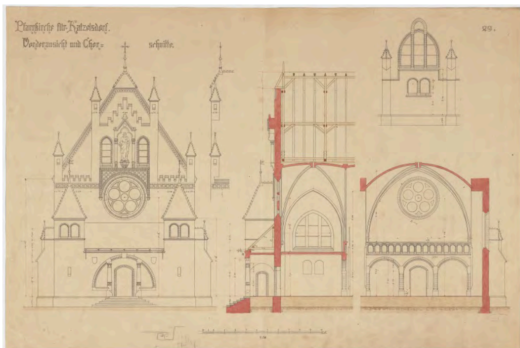
sign_6886 ... Pfarrkirche für Katzelsdorf. / 29. / Vorderansicht und Chorschnitte. / 1:50 / 1905 / realisierte Version
