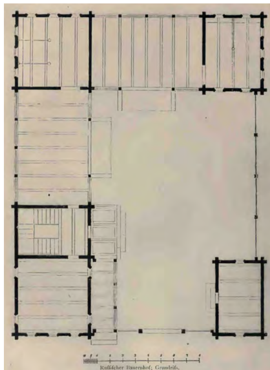
Russischer Bauernhof; Grundriss.
