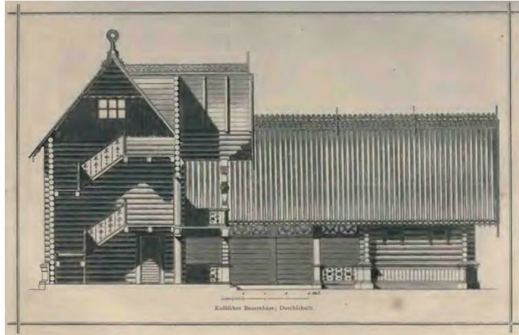
Russischer Bauernhof; Durchschnitt.
