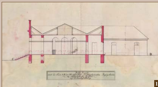
„Jery AB a CD loveckým zámekem knížky z Liechtensteina v Katzelsdorfském lese na panství Valtic“ od Josepha Korchaunda 5. dehes 1818. „Profil Ansicht nach der Linie AB und CD das Hochschloss des Liechtensteinischen Jagdschlusses im Katzelsdorfer Wald auf der Herrschaft Feldberg“ von Joseph Korchaund 5. April 1818.
