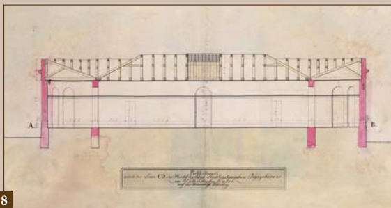
„Jery AB a CD loveckým zámekem knížky z Liechtensteina v Katzelsdorfském lese na panství Valtic“ od Josepha Korchaunda 5. dehes 1818. „Profil Ansicht nach der Linie AB und CD das Hochschloss des Liechtensteinischen Jagdschlusses im Katzelsdorfer Wald auf der Herrschaft Feldberg“ von Joseph Korchaund 5. April 1818.
